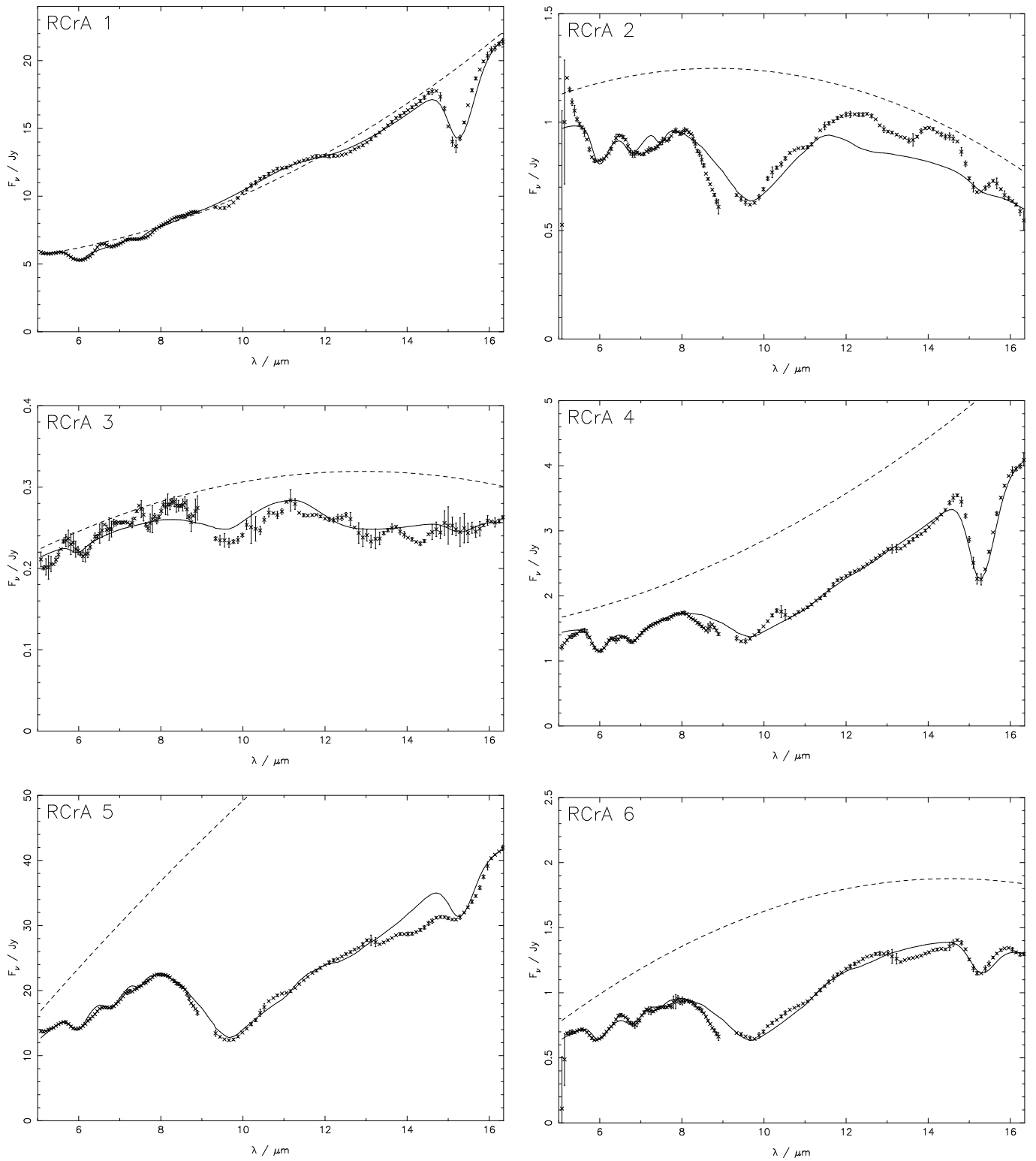
Fig. A.1. Spectra of RCrA 1-6.
